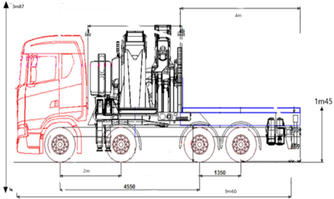
Schéma technique
